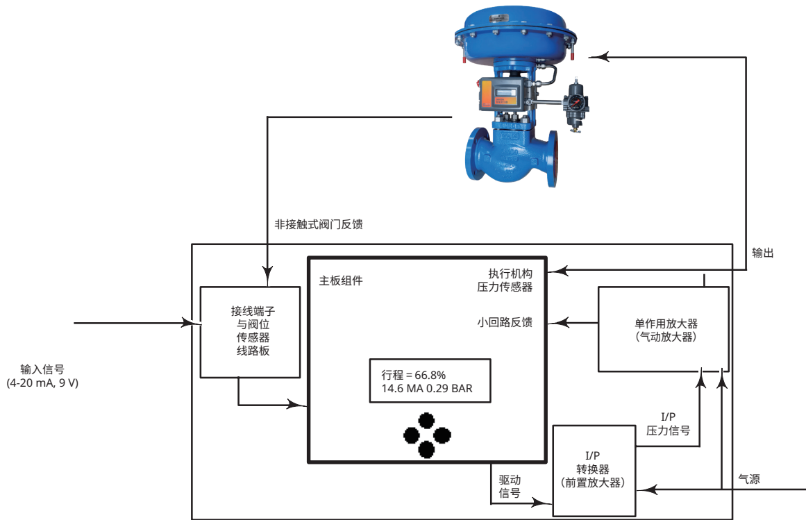
图 3 - GULDE 3800SA 智能定位器模块图
