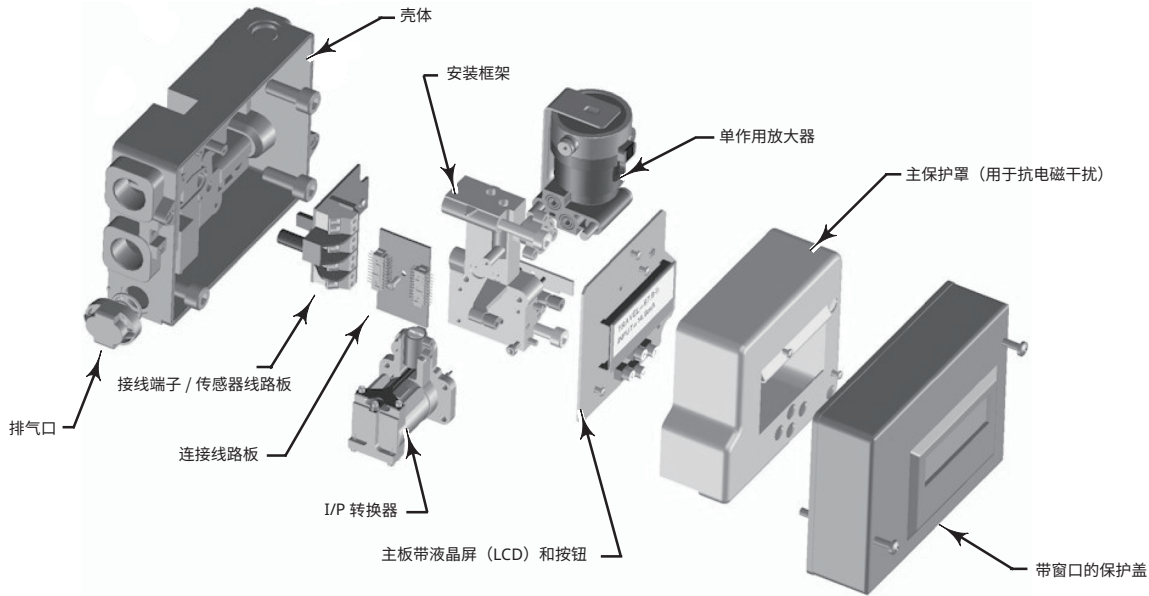
图 2 - GULDE 3800SA 智能定位器组件 (分解图)
