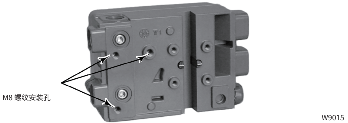
图 7. 线性执行机构的安装孔
