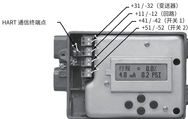
图 11. 回路、变送器和限位开关端子
