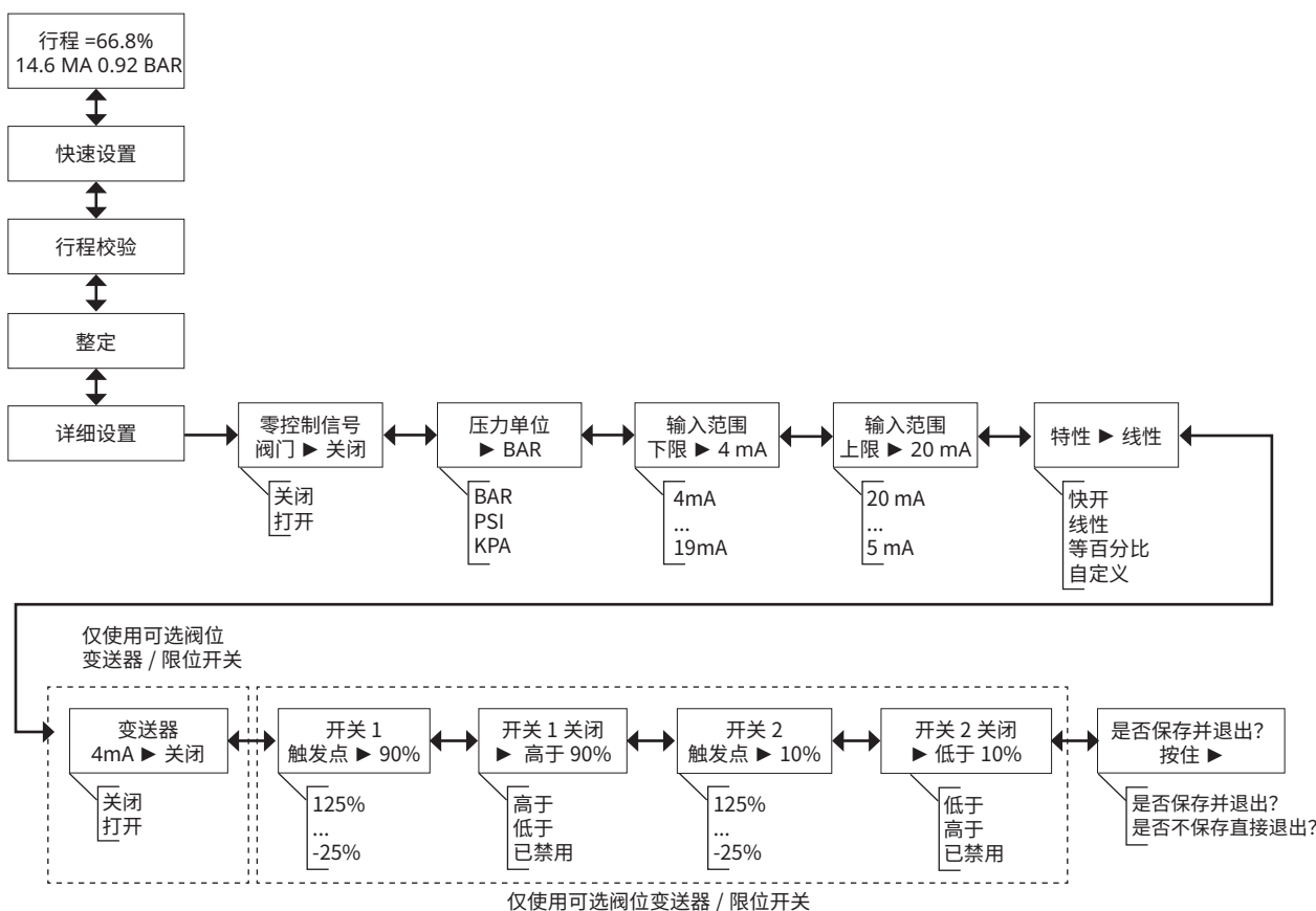
图 16. 详细设置流程图
