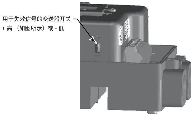
图 17. XMTR 开关
