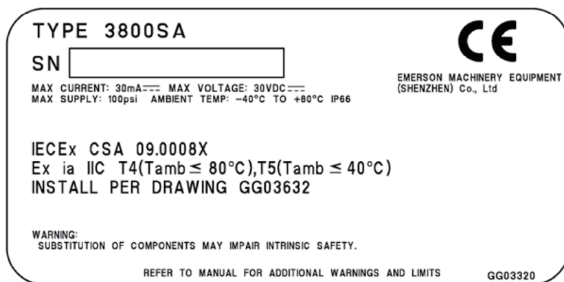
图 21. 典型的 IECEX 认证铭牌
