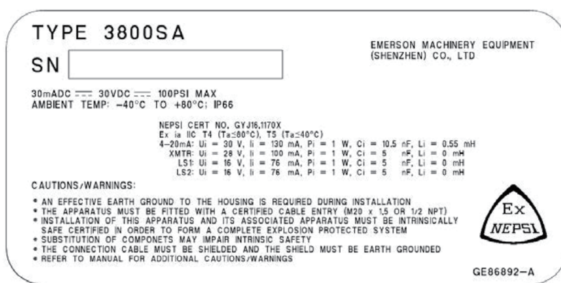
图 23. 典型的 NEPSI 认证铭牌
