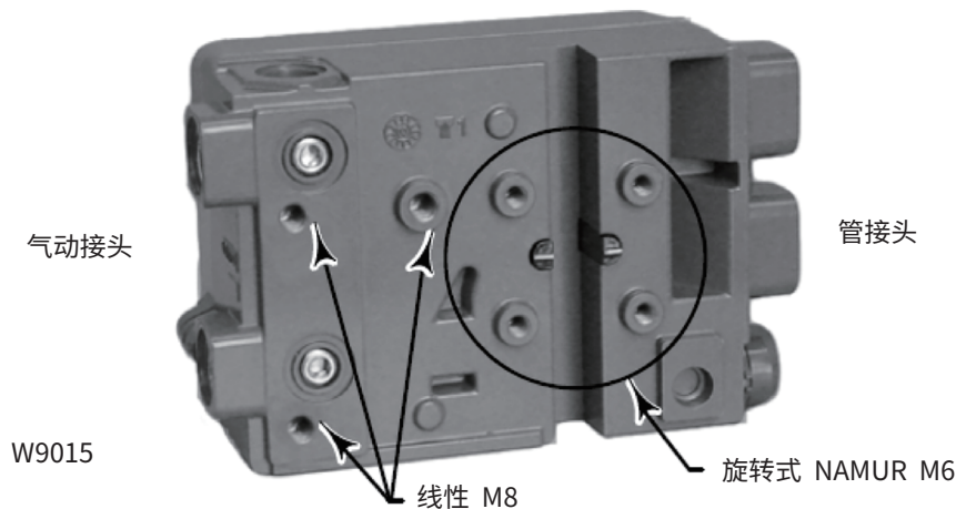
图 2. 不同类型的外壳
