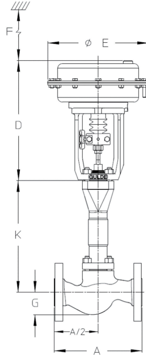
图 8- 5100 波纹管型尺寸图
