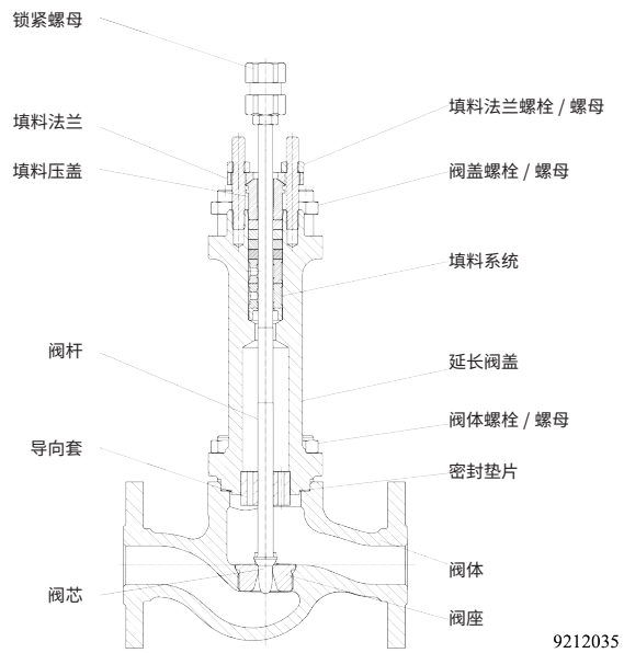
图 5- 延长型
