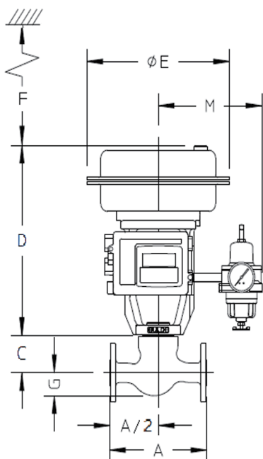
图 11-5100 阀门带定位器尺寸图
