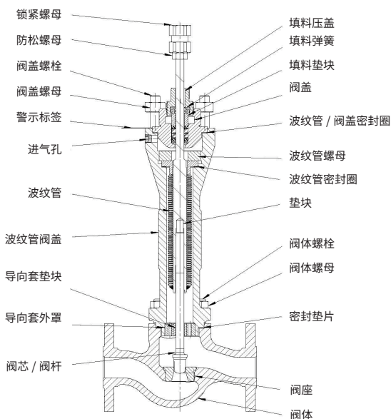
图 4- 波纹管型
