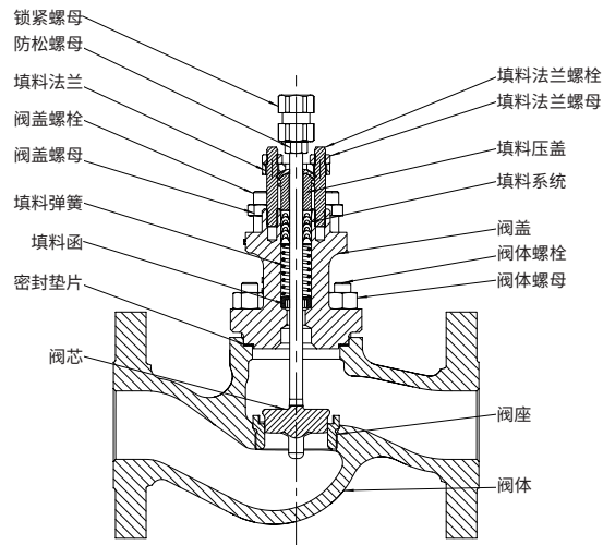
图 3- 独立阀盖型
