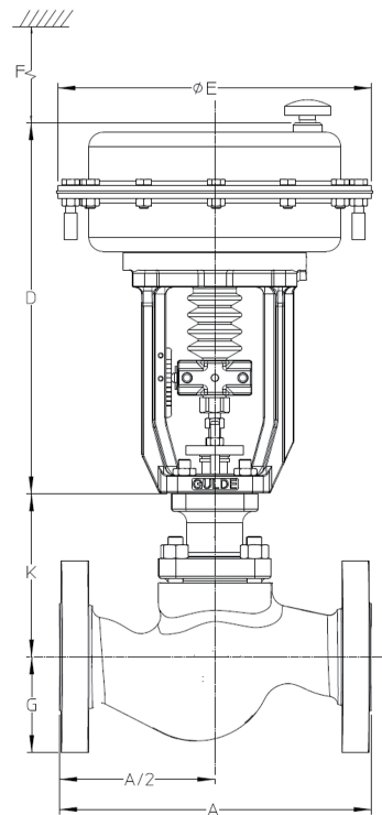
图 10- 5100 独立阀盖型尺寸图
