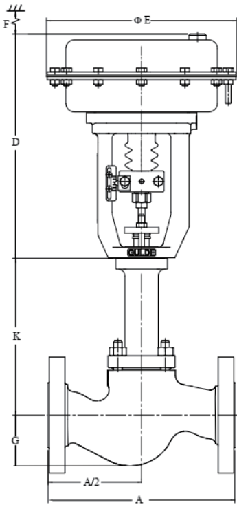
图 9- 5100 延长阀盖型尺寸图
