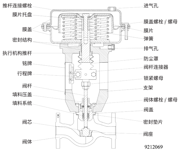
图 2- 标准型 + 执行机构
