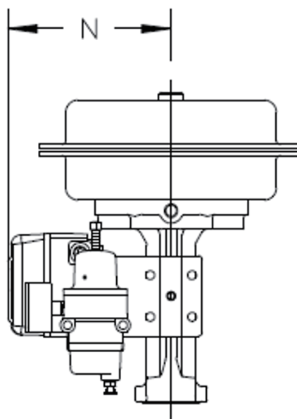
图 12-5100 阀门带定位器尺寸图
